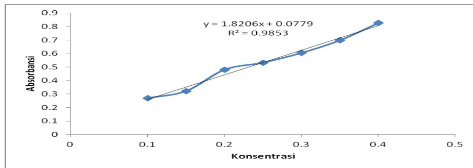
Gambar 1. Kurva baku yang diperoleh dari pengukuran absorbansi standar TMP (1,1,3,3 tetrametoksiopropana) yang diukur dengan spektrofometri sinar tampak pada panjang gelombang 532 nm.
